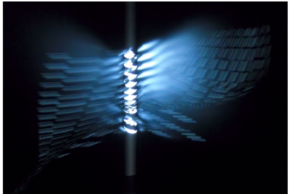
N-dimenzió 1
